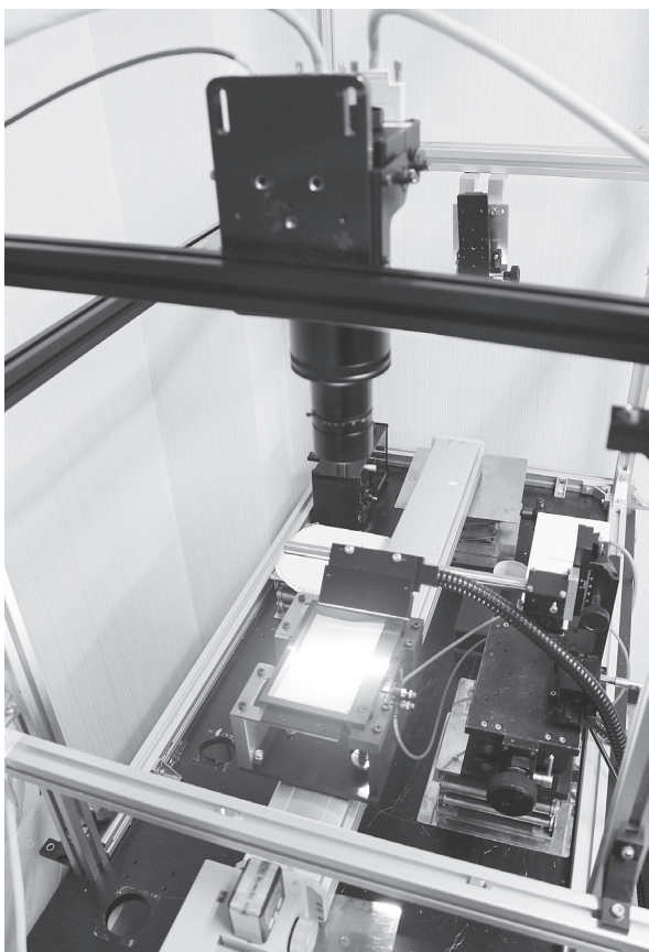
検査装置例。半導体チップをラインカメラで捉えて合否判定する。
